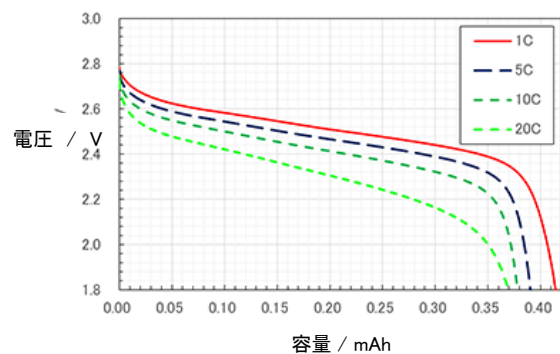
放電特性
