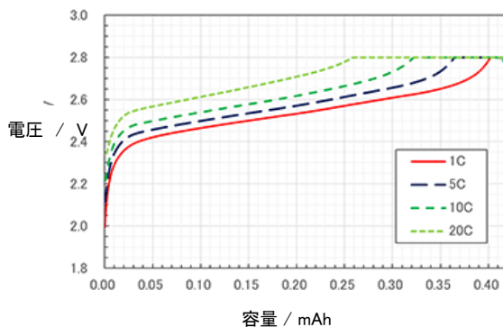
充電特性
